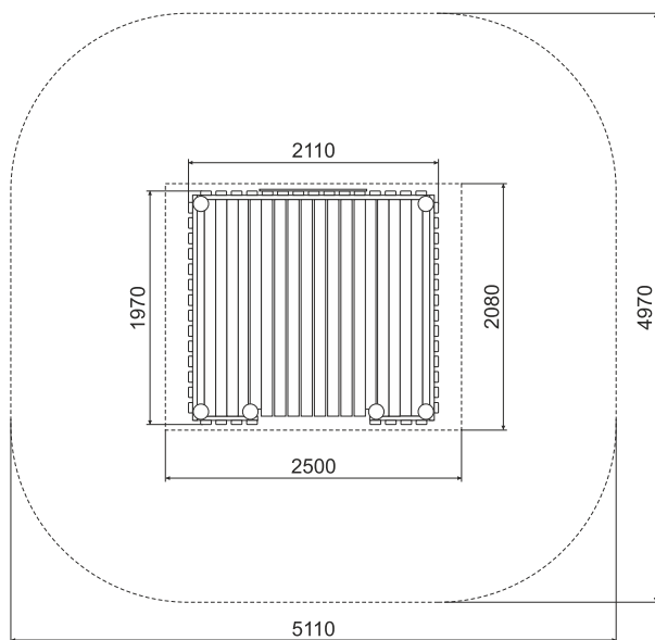
вид сверху
