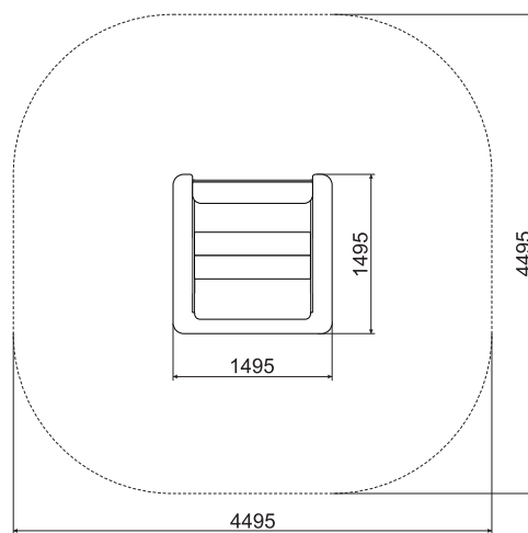
вид сверху
