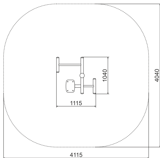
вид сверху
