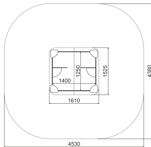
вид сверху
