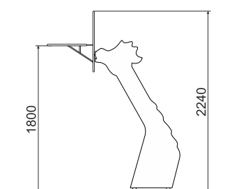
вид сбоку
