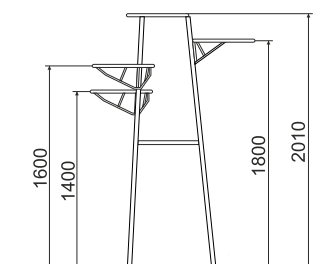
вид сбоку
